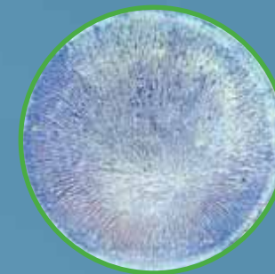
Cristallisation sensible eau Informée
