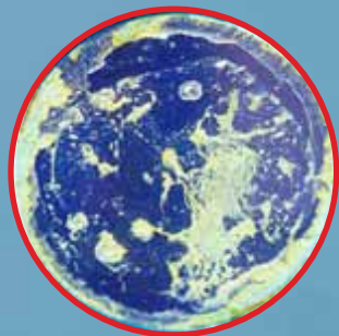
Cristallisation sensible eau du réseau
