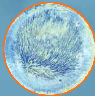
Cristallisation sensible eau dynamisée
